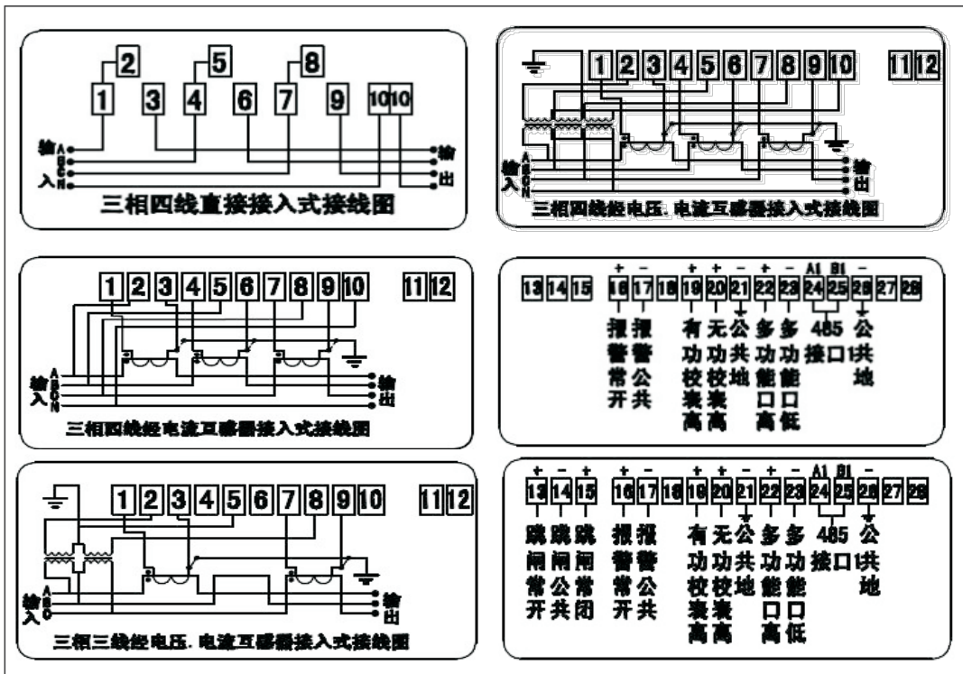
图3：主端子与功能端子接线图
