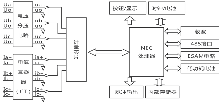
图1：电能表基本工作原理
