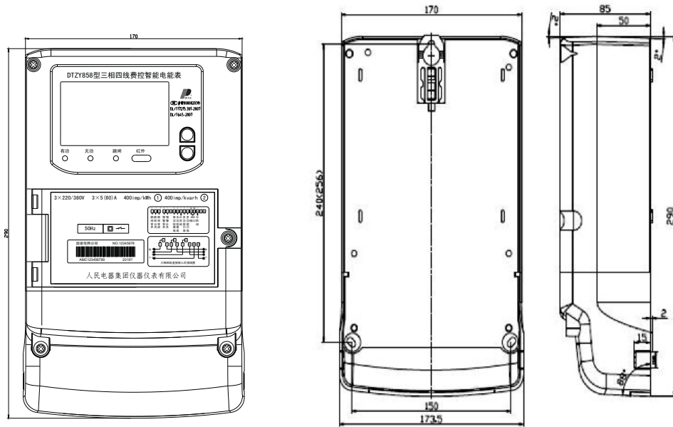
外形图
